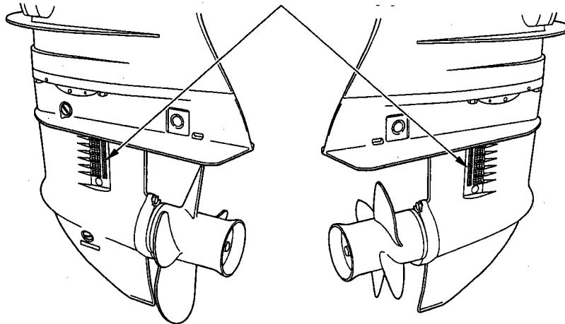
Jäähdytysveden ottoaukko
