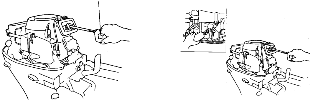
käynnistyskahva
