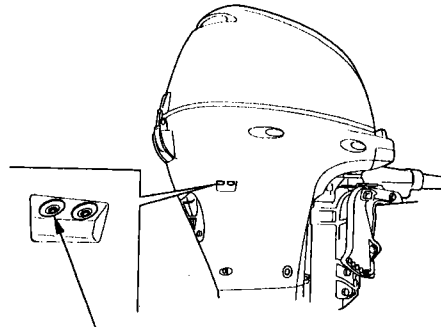
Jäähdytysveden tarkistusaukko
