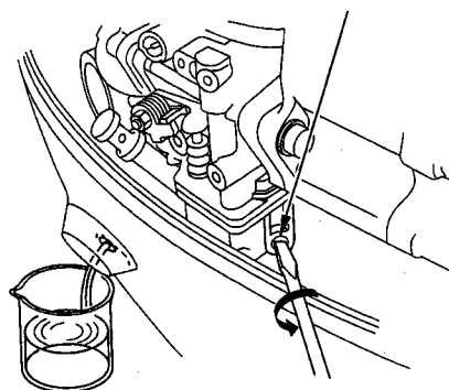
Tyhjennysruuvi
